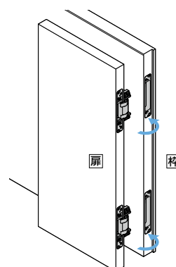
旗丁番は軸がでっぱり外側から見えてしまう
