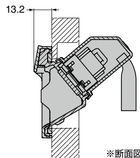
カバーの部品 + コンセントのセット (組立後イメージ)
