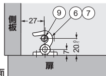
図4 B-B断面
