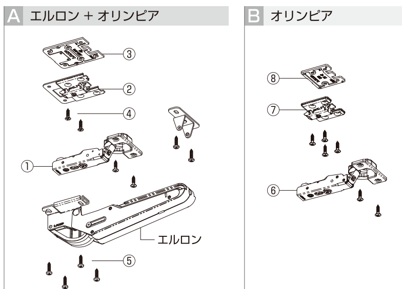
ARN-3型(上開き仕様)の場合
