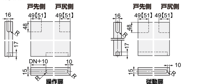
扉厚36 mm、上レール(面付用)使用時
