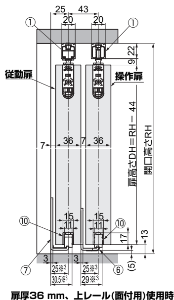
扉厚36 mm、上レール(面付用)使用時
