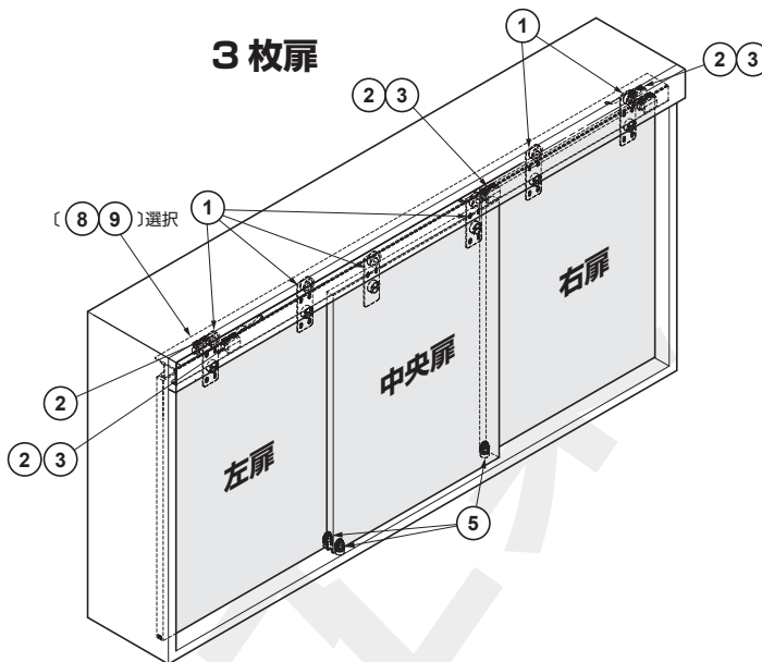
図は、中央扉が左側に開く場合を示します。
