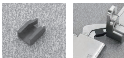
⑥ 92°開き止めパーツ 品番: SSEL637X3 (開き角度を105°から92°に制限します)
