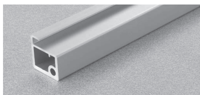
③ アルミフレーム(26mm厚、適応ガラス厚:4mm) 品番: SDEL6LP300P(ニッケル色) 品番: SDEL6LP300T(チタン色) 品番: SDEL6LP300W(ホワイト) 品番: SDEL6LP300B(ブラック)
