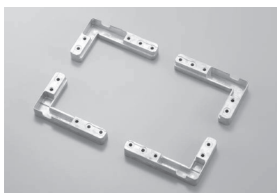
② コーナーコネクター 品番: SDEL6BSFV02
