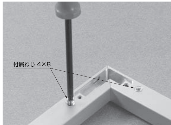
【2】コーナーコネクタをねじ止め
