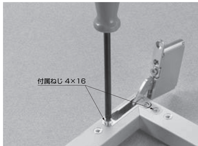
【4】丁番をねじ止め
