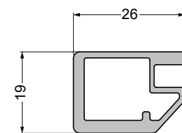
④ アルミフレーム(19mm厚、適応ガラス厚:4mm) 品番: SDEL9LP300P(ニッケル色) 品番: SDEL9LP300T(チタン色) 品番: SDEL9LP300W(ホワイト) 品番: SDEL9LP300B(ブラック)
