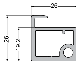
③ アルミフレーム(26mm厚、適応ガラス厚:4mm) 品番: SDEL6LP300P(ニッケル色) 品番: SDEL6LP300T(チタン色) 品番: SDEL6LP300W(ホワイト) 品番: SDEL6LP300B(ブラック)
