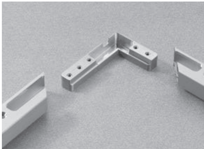
【1】コーナーコネクタをアルミフレームに挿入
