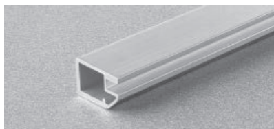
④ アルミフレーム(19mm厚、適応ガラス厚:4mm) 品番: SDEL9LP300P(ニッケル色) 品番: SDEL9LP300T(チタン色) 品番: SDEL9LP300W(ホワイト) 品番: SDEL9LP300B(ブラック)
