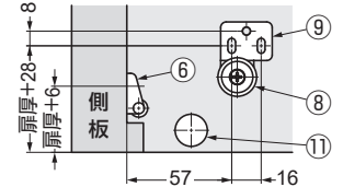
視イ (ブラケット取付の場合)
