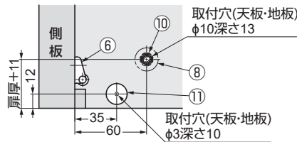
視イ (インサート取付の場合)
