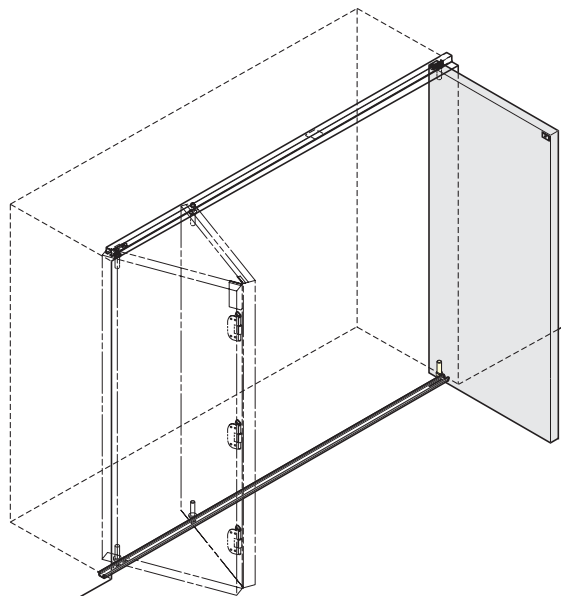
上記は、ピボット式折戸 FD30-F 下レール仕様 吊元固定用 (2点鎖線部) 品番：FD30FAP との組み合わせ例です。
