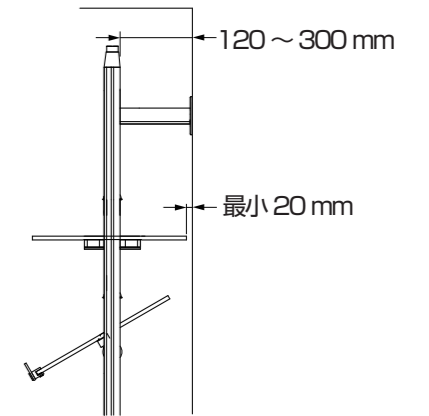
壁固定座縦フレームカットタイプ XL-US02-S009 の時は使用する長さによって 穴加工をオフセットする必要があります。
