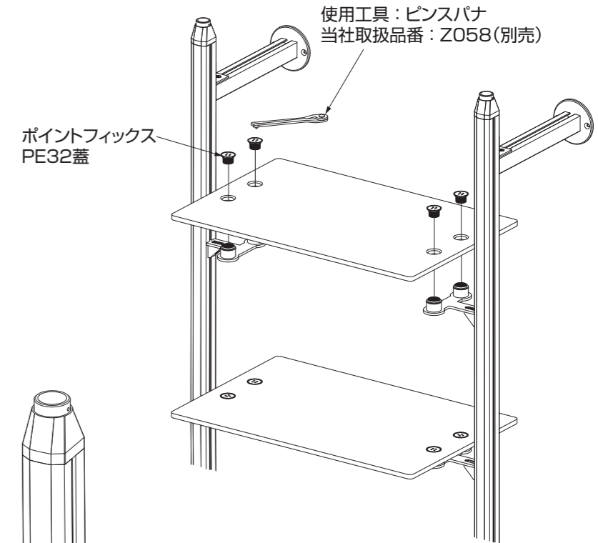
壁固定座2本ロッドタイプ XL-US02-S008 の時は穴加工を オフセットする必要があります。 X寸法：70mm
